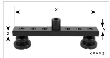
SP010-63-002 185\text{mm} \times 30\text{mm} \times 13\text{mm}
